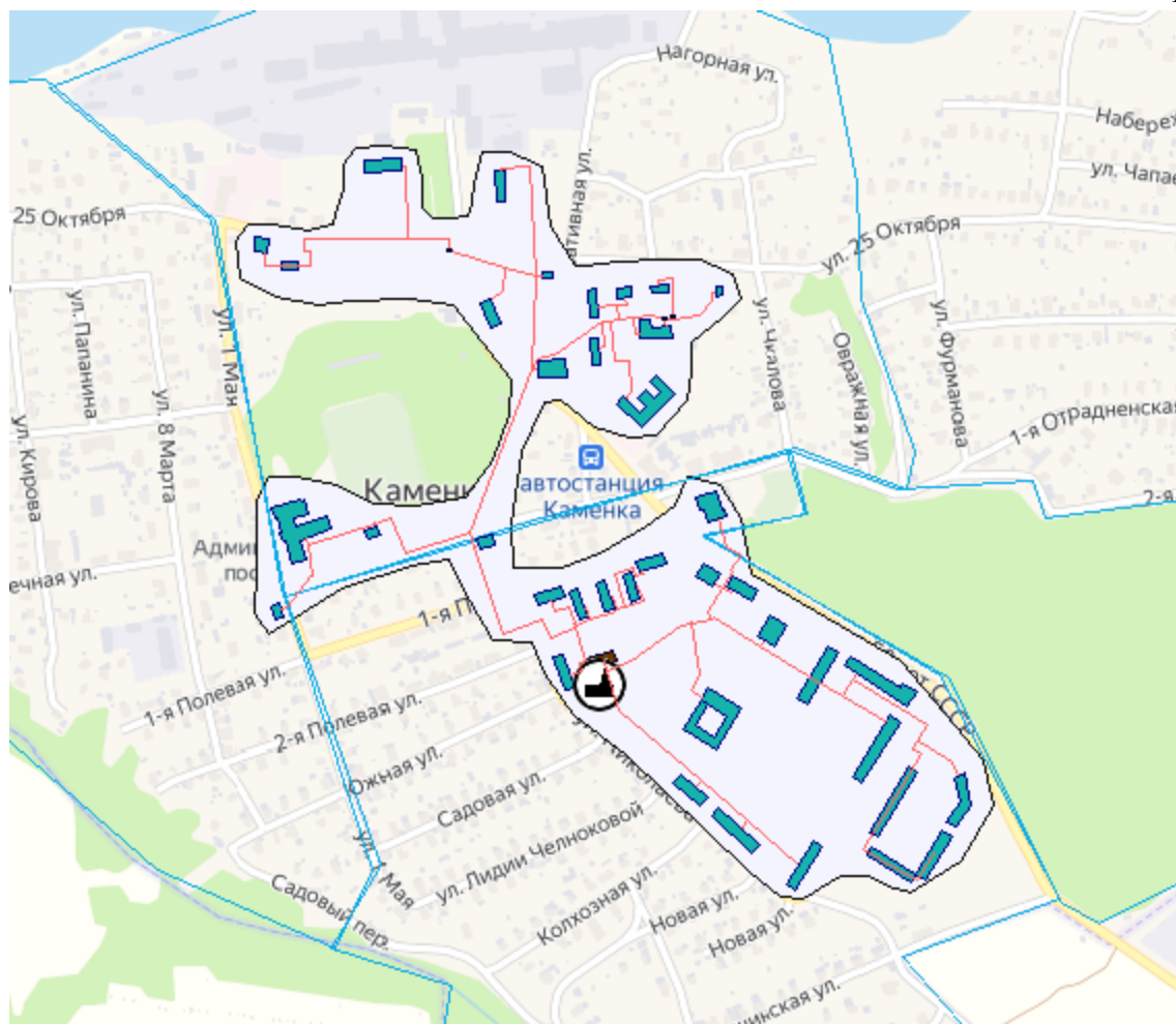
Присоединенная нагрузка в зоне действия источников
